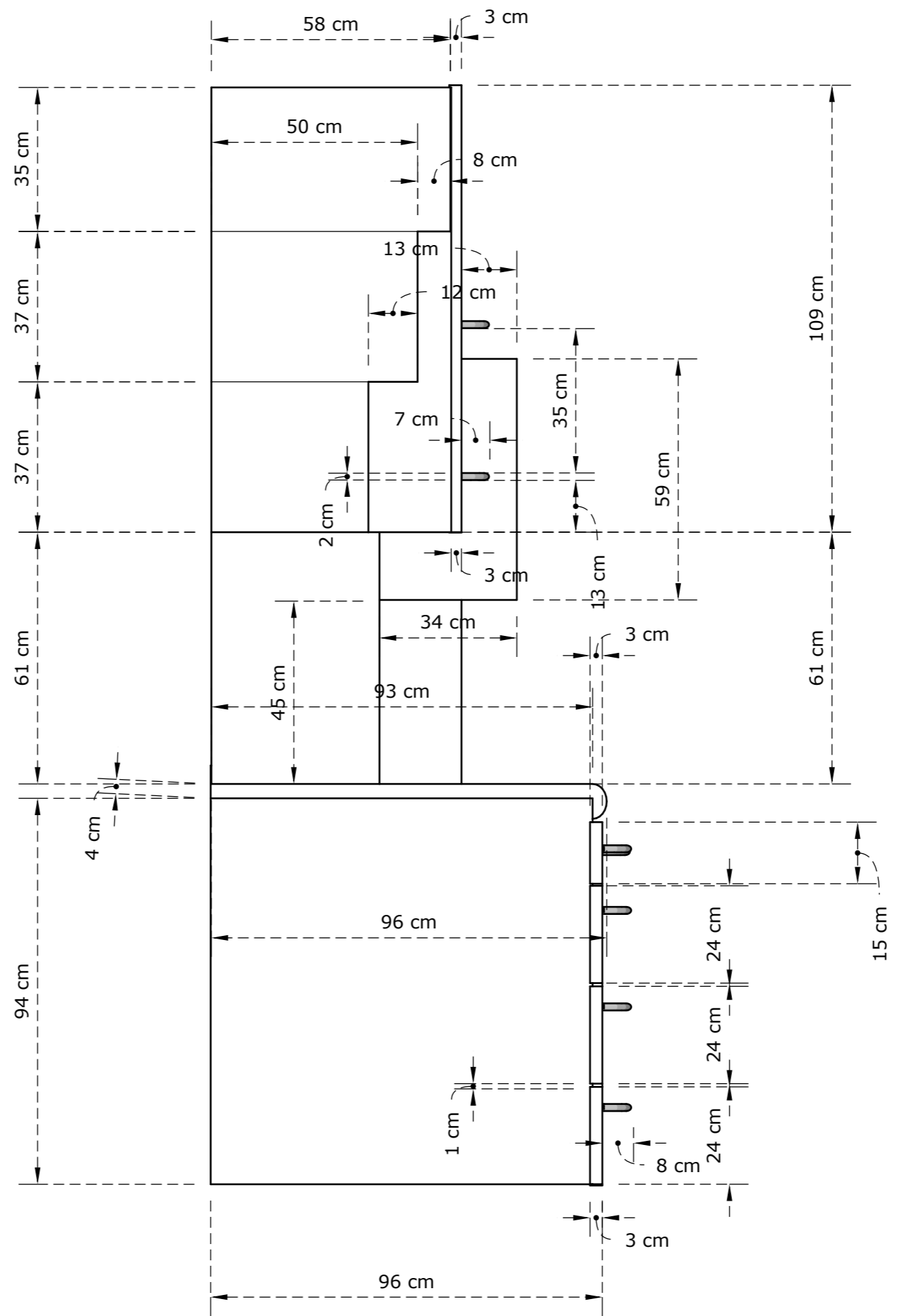
VISTA LATERAL
