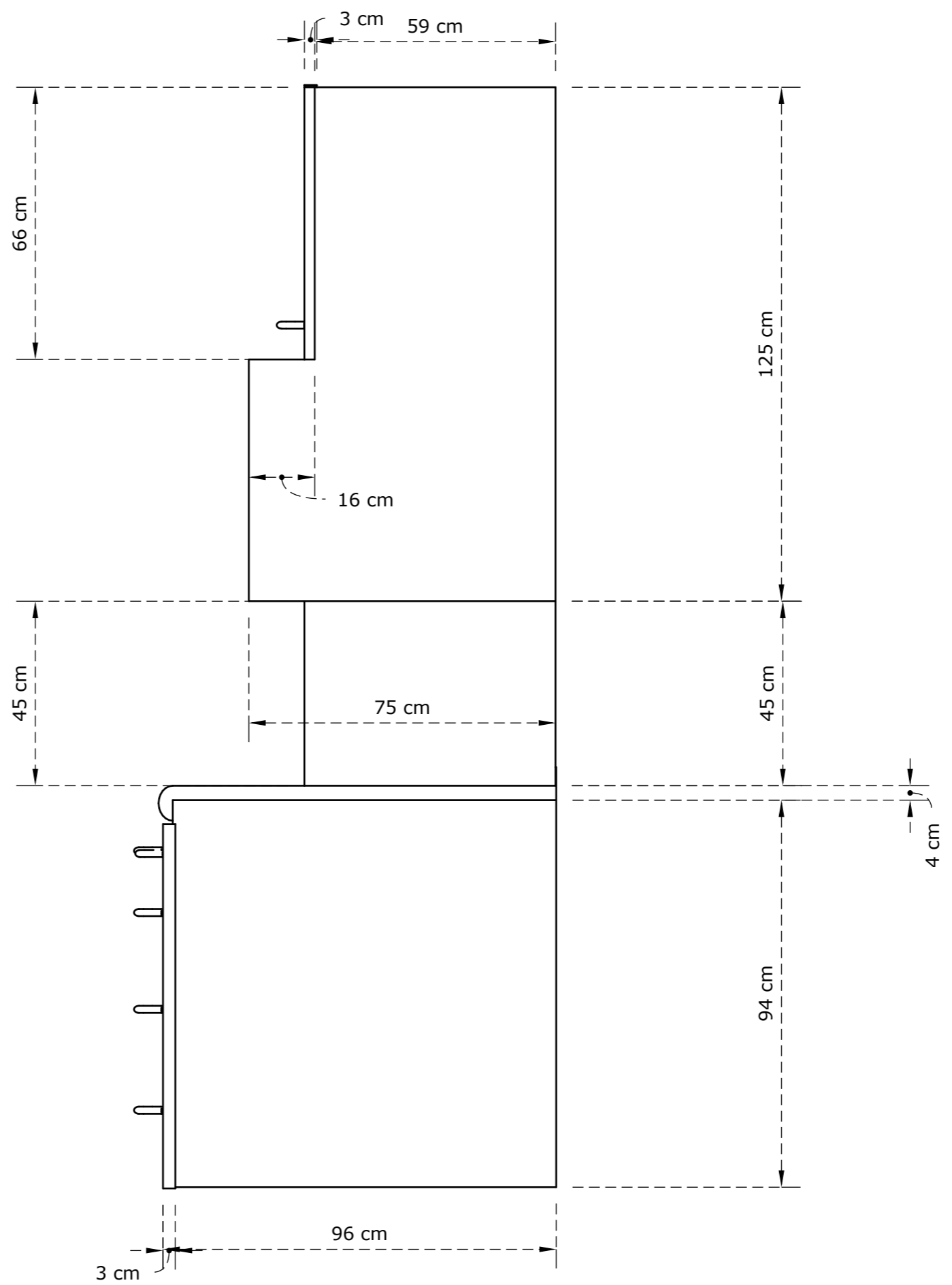
VISTA LATERAL
